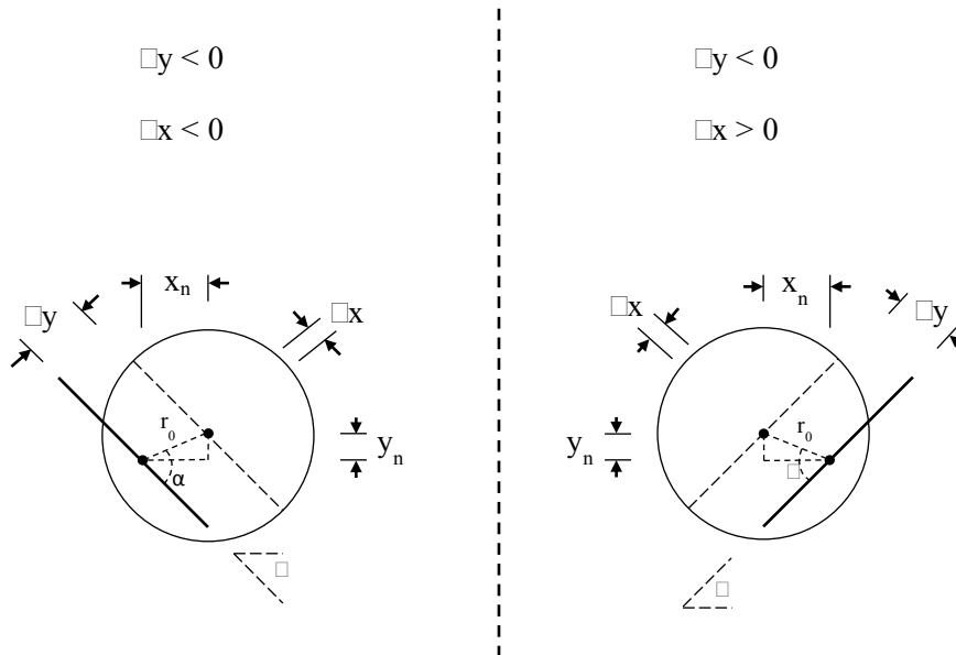
Fig. 3. Offset coordinates
